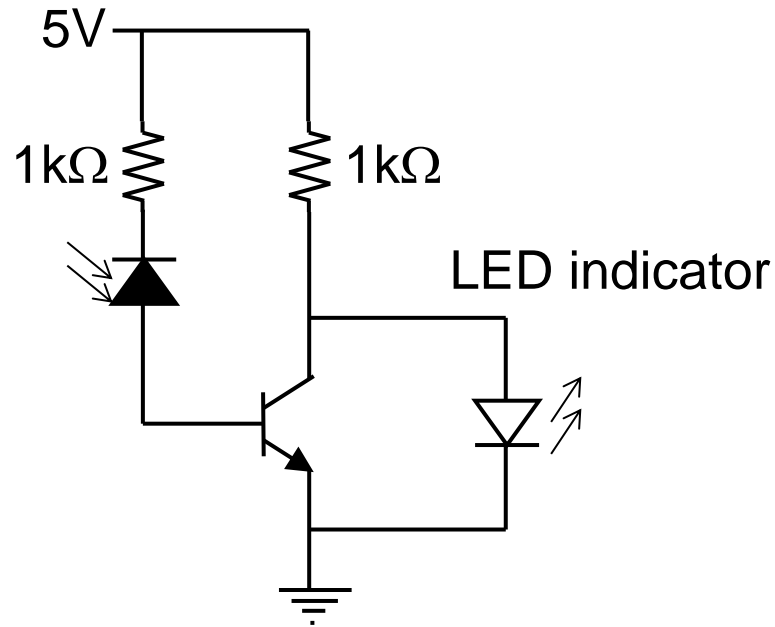
Infra-red detector
